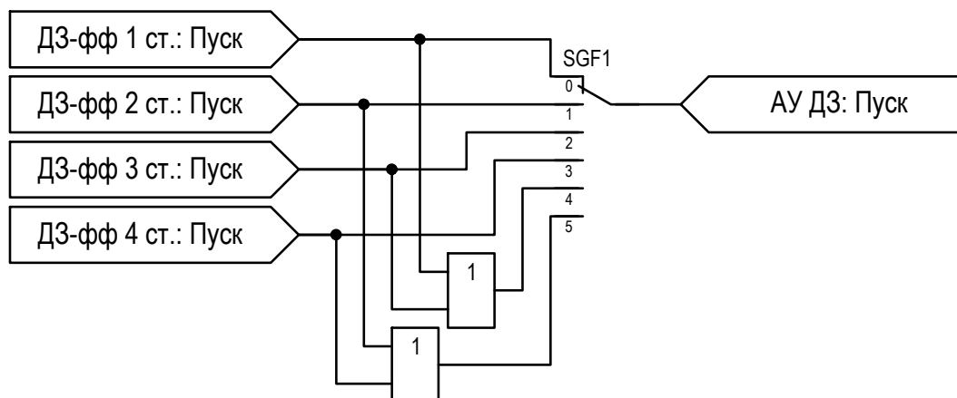
Рисунок 2.8 – Функциональная схема «АУ Д3»
